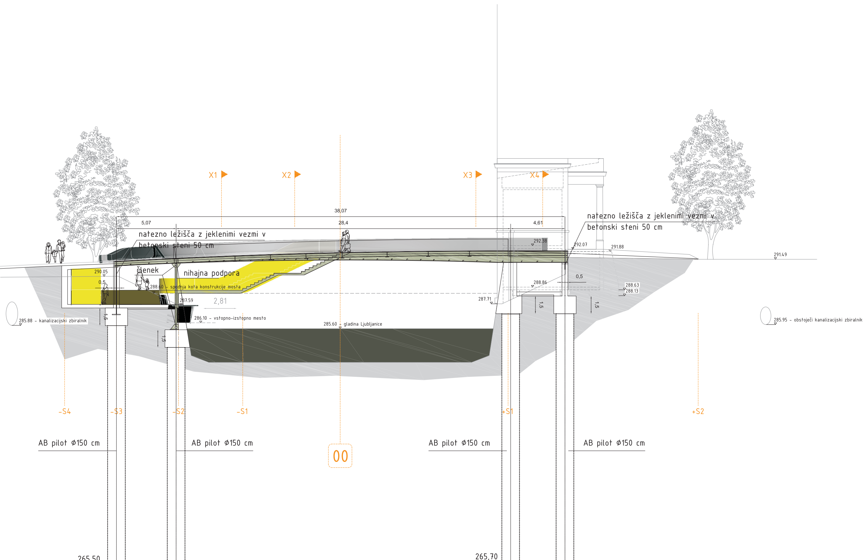
↑ VZDOLŽNA FASADA Z NOSILNO KONSTRUKCIJO
